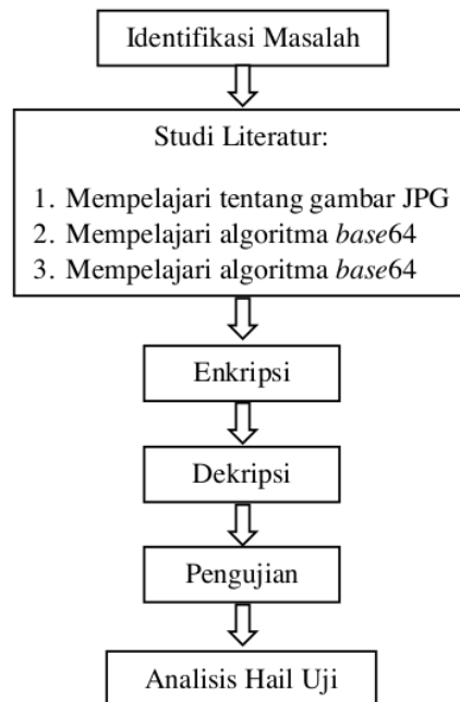
Gambar 1 Desain Penelitian
