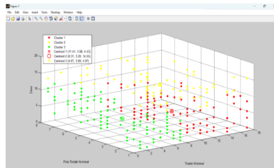
Gambar 4.3 Grafik Hasil Pengujian
