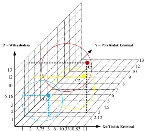
Gambar 3. 1 Grafik Cluster berdasarkan perhitungan yang telah dilakukan
