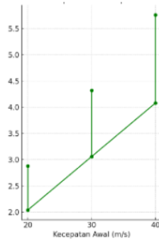
Waktu Tempuh vs Kecepatan Awal: Grafik ini menunjukkan waktu yang dibutuhkan untuk mencapai jarak horizontal pada berbagai kecepatan awal
