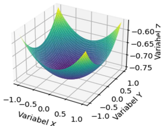
Gambar 2 Grafik Persamaan 16 - x^2 - y^2
