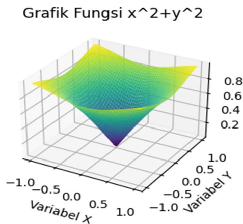
Gambar 1 Grafik Persamaan x^2 + y^2
