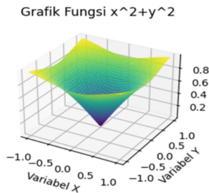
Gambar 1 Grafik Persamaan x^2 + y^2
