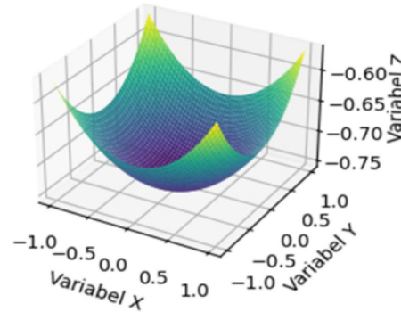
Gambar 2 Grafik Persamaan 16 - x^2 - y^2
